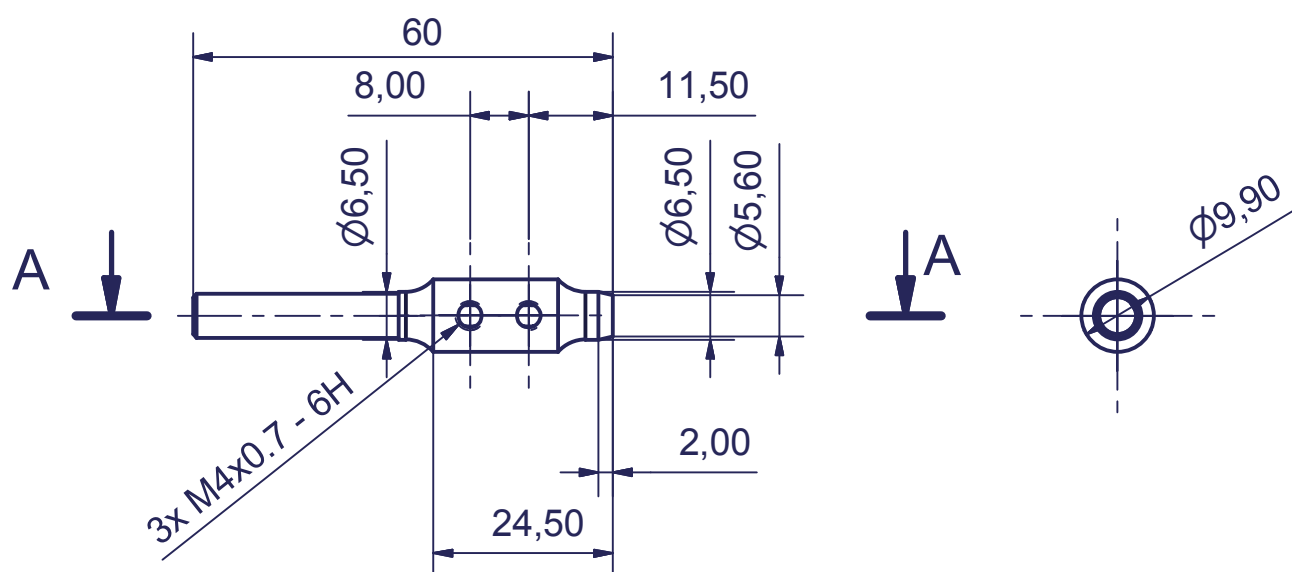
A-A ( 1 : 1 )
