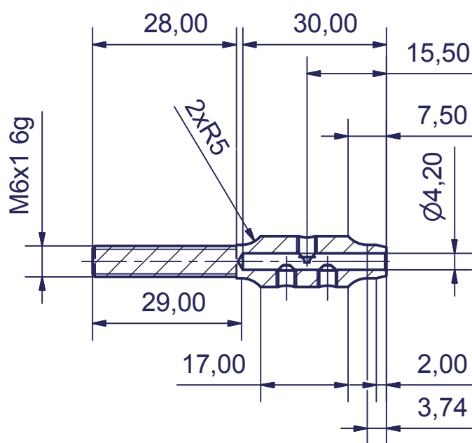
A-A ( 1 : 1 )
